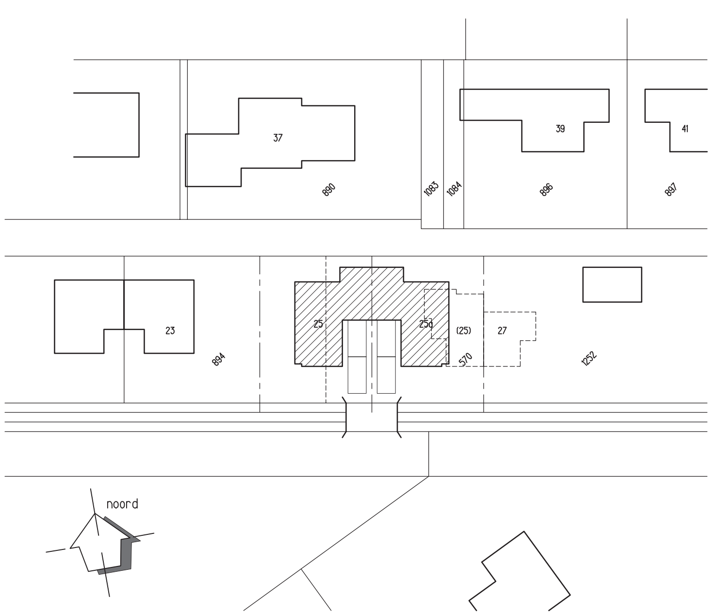
situatie
