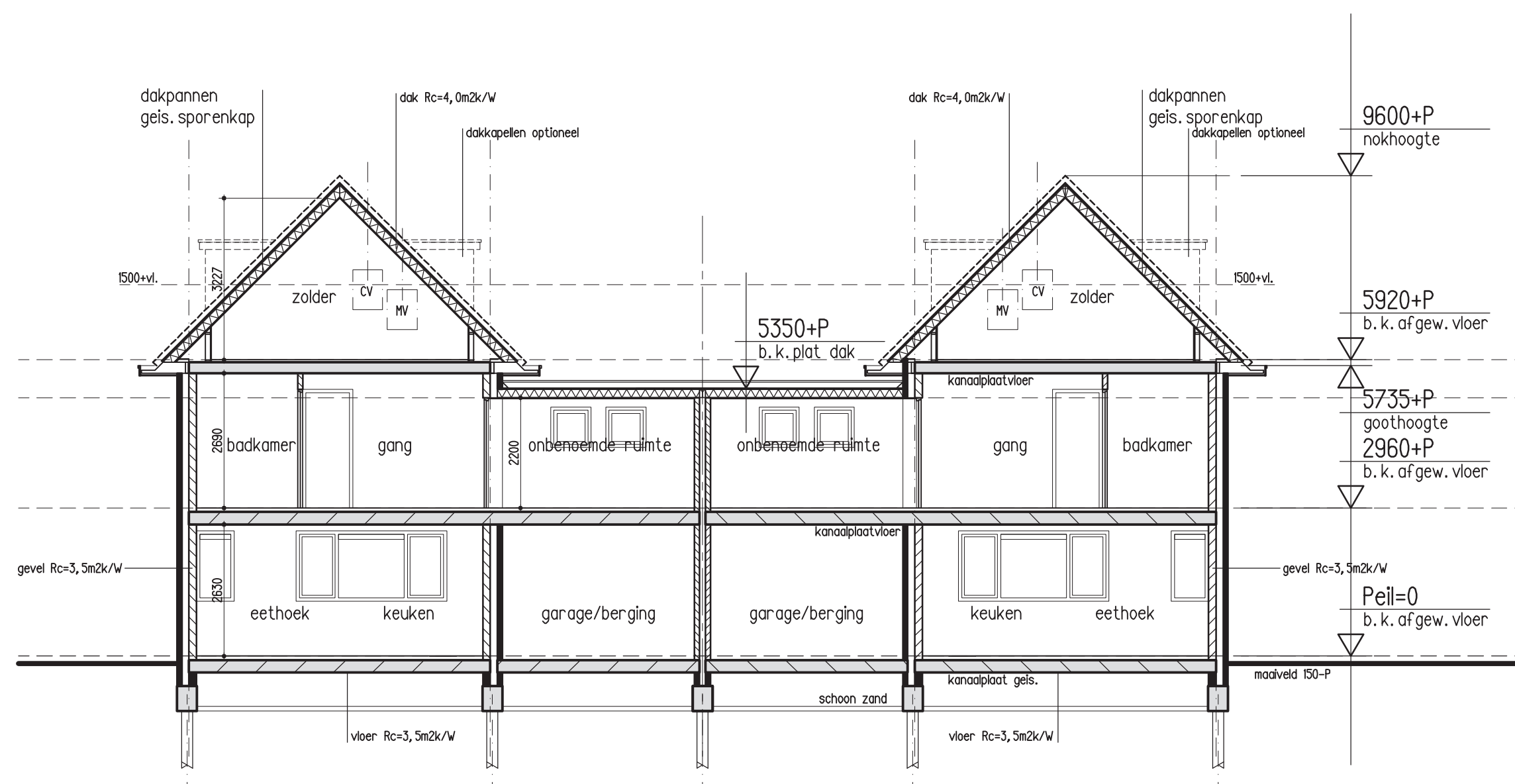
doorsnede A-A
