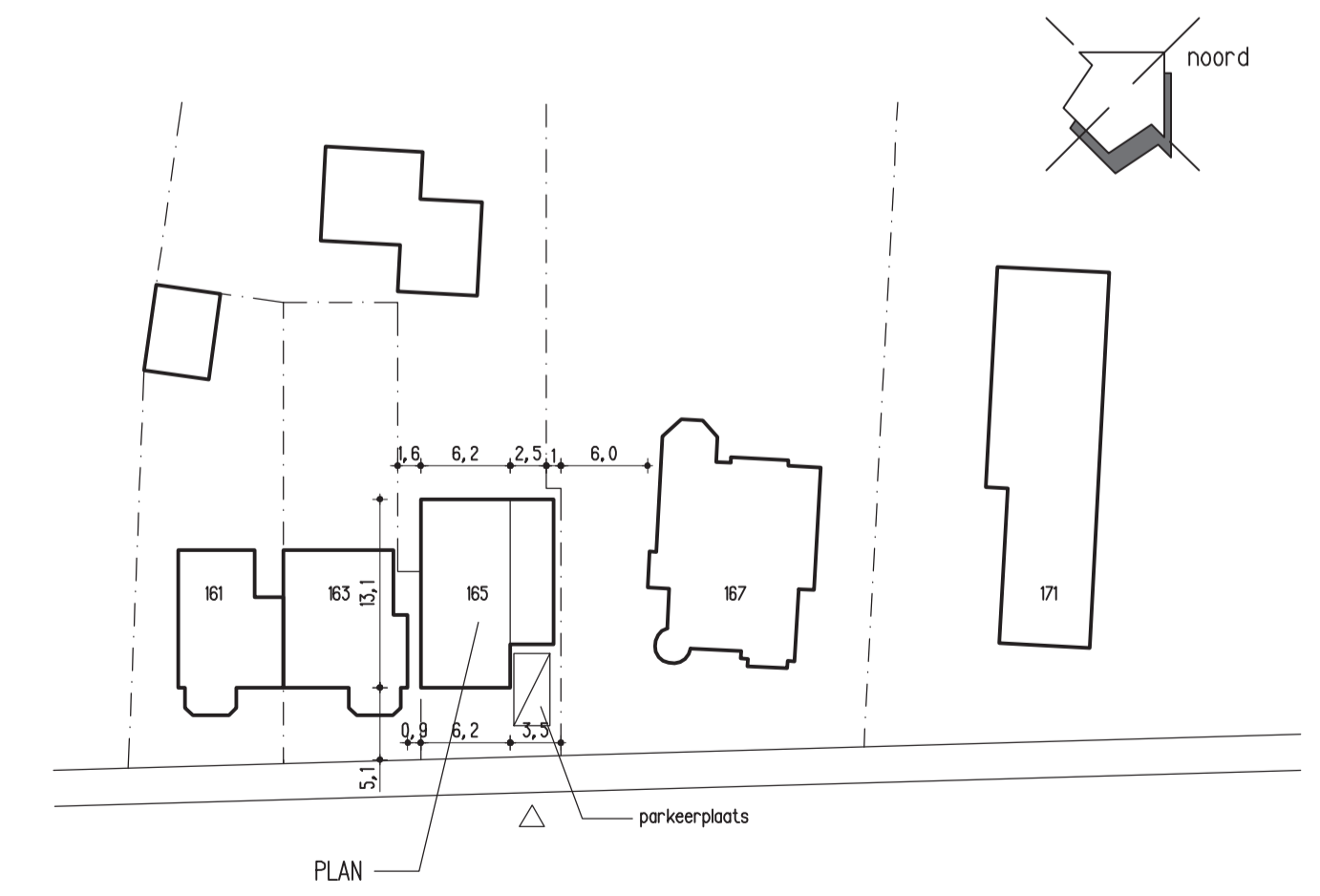
situatie
