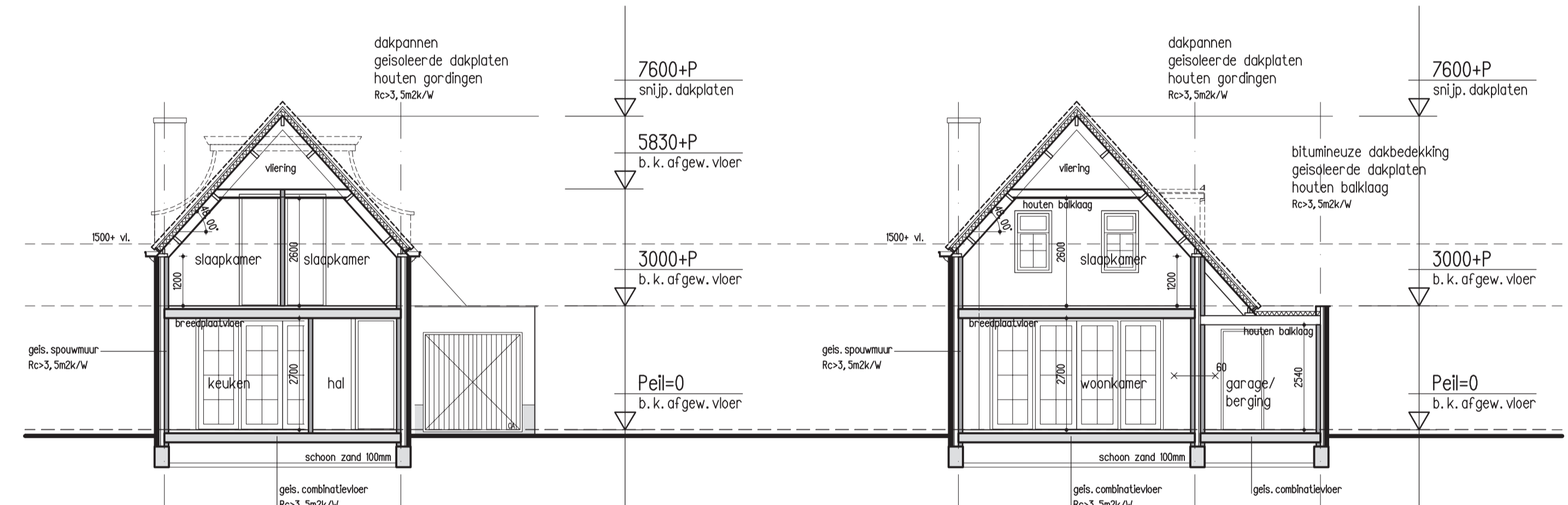
doorsnede A-A
